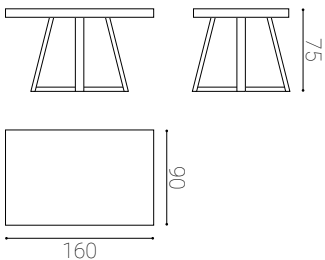
Ref. N7063 Opciones medidas de mesa: 120 x 90 x 75 cm / 140 x 90 x 75 cm / 160 x 90 x 75 cm / 190 x 90 x 75 cm / Medidas del dibujo técnico según fotografía. Puntos totales según dibujo técnico: 396 pt Materiales composición: Roble brown, Beige.
